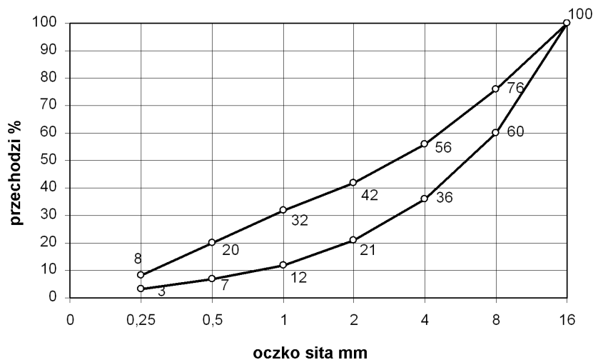
Rys. 1. Graniczne krzywe uziarnienia kruszywa 0 ÷ 16 mm
