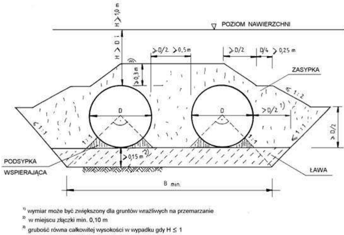
Rys. 9. Zasyпка nad przepustem dwururowym
