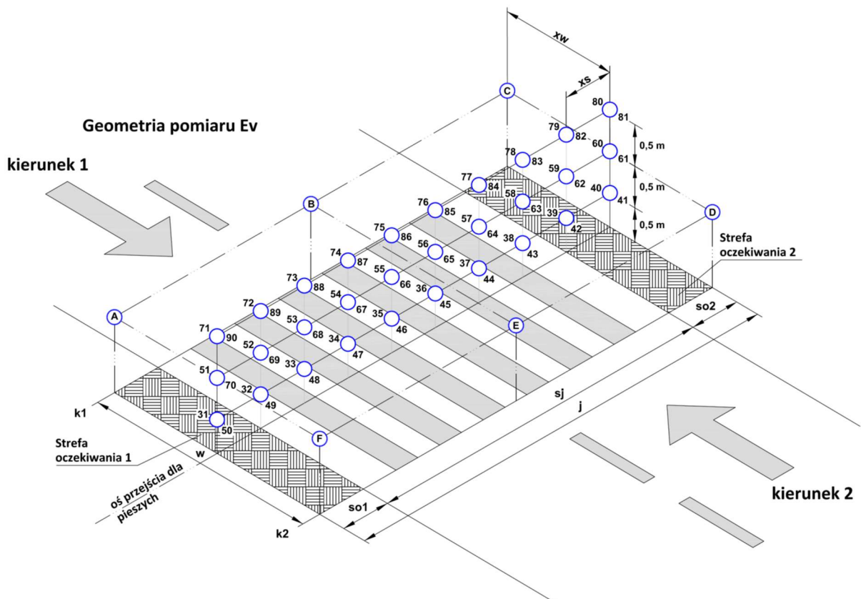
Rys. 6.3.1. Schemat siatki punktów do pomiaru natężenia oświetlenia niezbędnego do określenia klasy oświetleniowej PC (oświetlenie dedykowane) oświetlenia w płaszczyźnie pionowej ( E_v ) na przejściu dla pieszych
