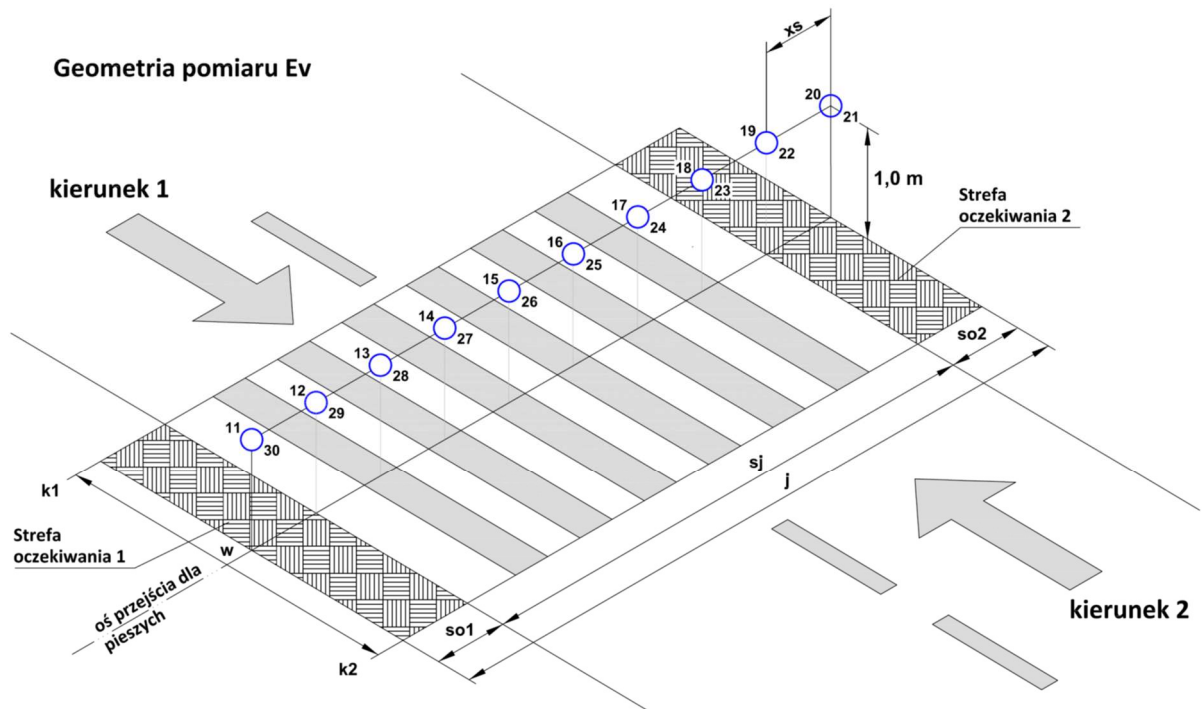
Rys. 8.4.1. Przykładowe rozmieszczenie punktów pomiarowych natężenia oświetlenia w płaszczyźnie pionowej ( E_v ) na przejściu dla pieszych stosowana w procedurze kontrolnej
