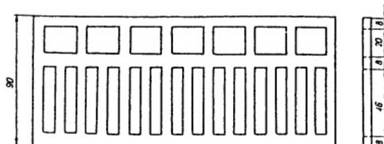
Deska ażurowa kombinowana 202 x 90 x 5 cm
