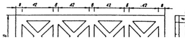
Deska ażurowa krzyżulcowa 202 x 60 x 5 cm
