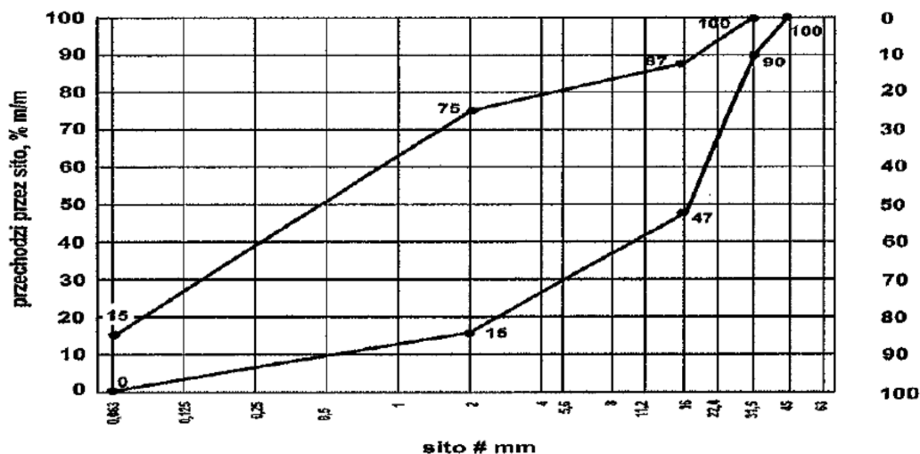
Mieszanka niezwiązana 0/31,5 do nawierzchni z kruszywa niezwiązanego
