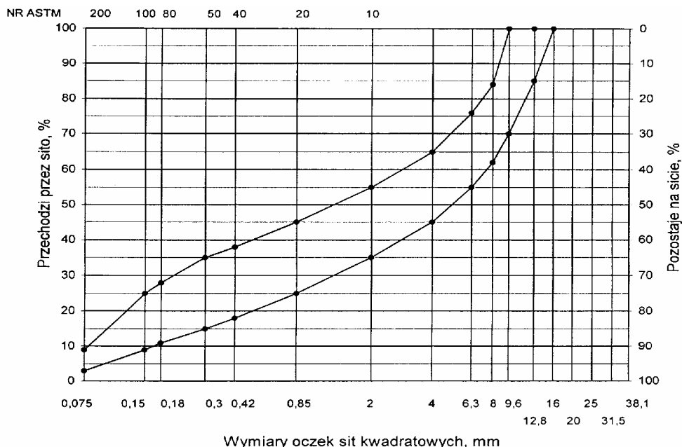
Rys. 3. Krzywe graniczne uziarnienia mieszanki mineralnej BA od 0 do 12,8 mm do warstwy wyrównawczej nawierzchni drogi o obciążeniu ruchem KR1 lub KR2
