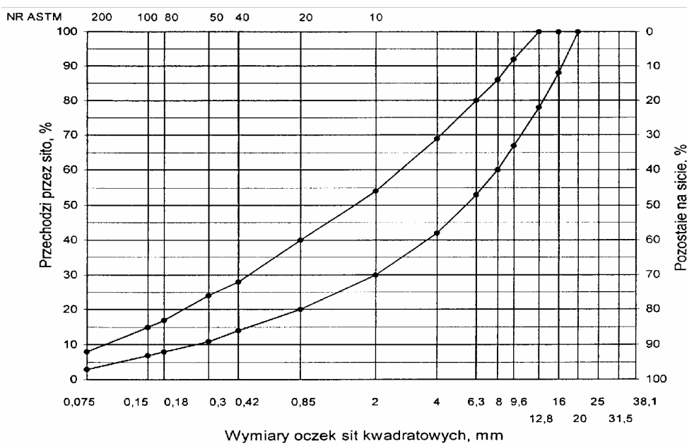
Rys. 2. Krzywe graniczne uziarnienia mieszanki mineralnej BA od 0 do 16 mm do warstwy wyrównawczej nawierzchni drogi o obciążeniu ruchem KR1 lub KR2
