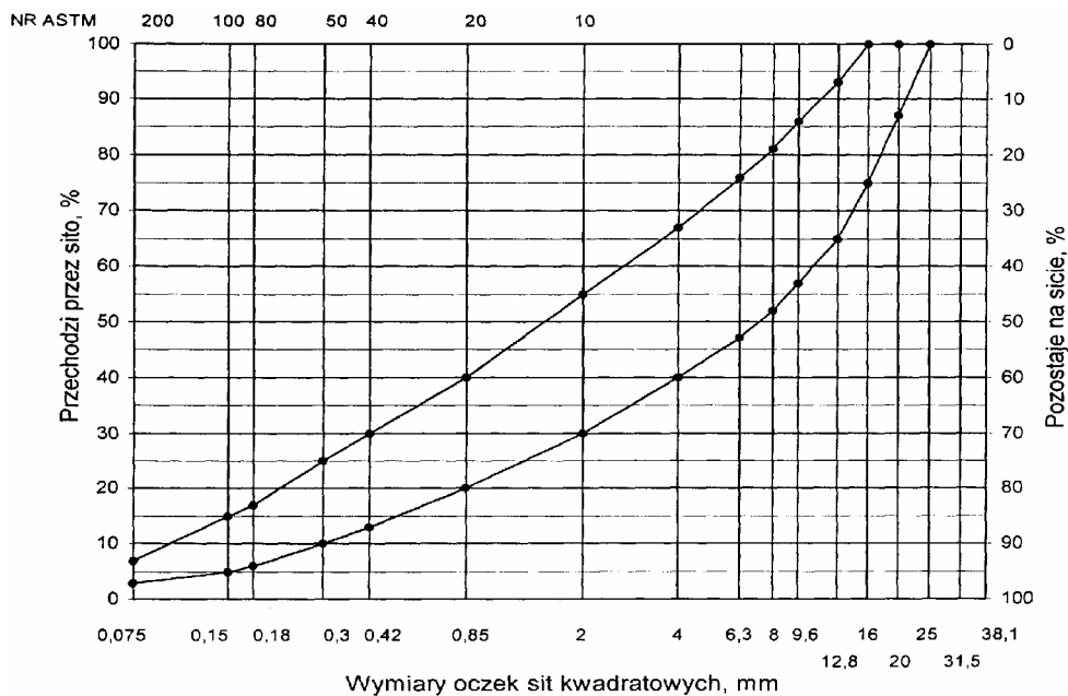
Rys. 1. Krzywe graniczne uziarnienia mieszanki mineralnej BA od 0 do 20 mm do warstwy wyrównawczej nawierzchni drogi o obciążeniu ruchem KR1 lub KR2
